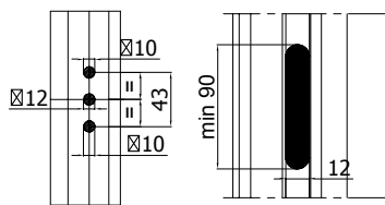
ГЛУБИНА СВЕРЛЕНИЯ 47 мм / PERFORATION DEPTH 47mm
