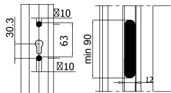
ГЛУБИНА СВЕРЛЕНИЯ 52 мм / PERFORATION DEPTH 52mm
